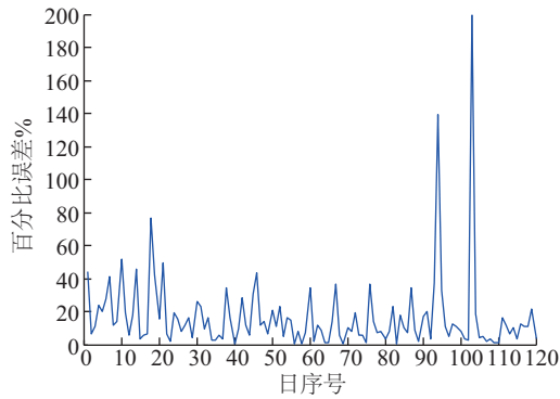
图4 福山站GRNN网络预估百分比误差
